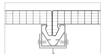
Spessore 8-20-32
